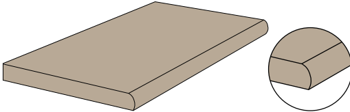
30x60,4 - 12"x24" ≠ 20 mm Elemento Bordo Becco - Half bullnose element Element mit Eckabrundung - Élément arrondi à 1/4 Esterno Rettificato 2LU61BB Ivoire 2LU62BB Crème 2LU63BB Doré
