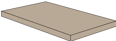
33x61,4x5 - 13"x24"x2" DX Angolare ad Elle - L-shaped Corner Element L-Form ECKelement - Élément d'angle en "L" Naturale LU1GAD Ivoire LU2GAD Crème LU3GAD Doré Esterno LU1GADE Ivoire LU2GADE Crème LU3GADE Doré
