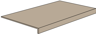
33x61,4x5 - 13"x24"x2" Lineare ad Elle - L-shaped Element L-Form Element - Élément linéaire en "L" Naturale LU1GL Ivoire LU2GL Crème LU3GL Doré Esterno LU1GLE Ivoire LU2GLE Crème LU3GLE Doré
