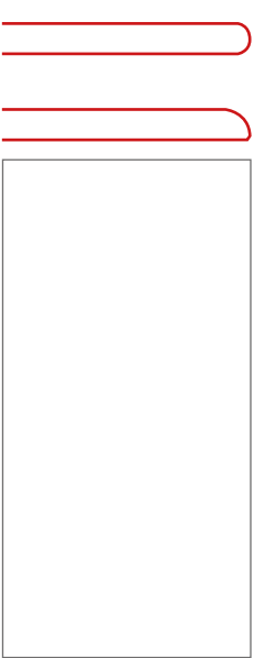
Bordo Tondo - Fully rounded edge Runde Kante - Bord Rond Bordo Becco - Semi-rounded edge Eingekerbte Kante - Bord Arrondi
